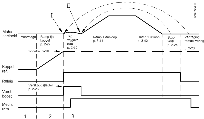
Afbeelding 3.4: Remvrijgaveprocedure voor mechanische rembesturing bij hijstoepassingen
