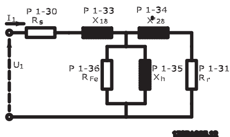
Afbeelding 3.1: Motorequivalentiediagram voor een asynchrone motor
