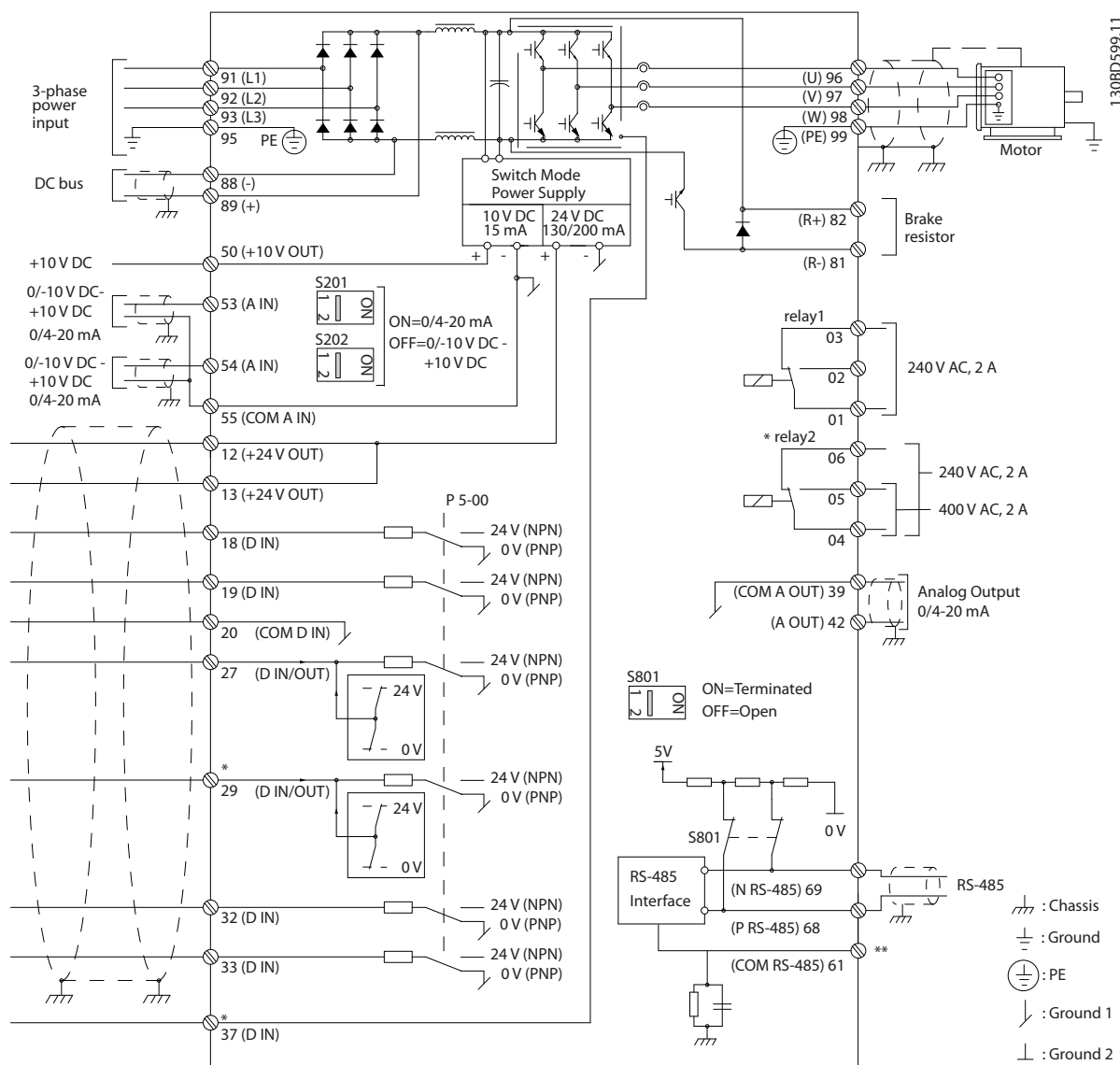
Afbeelding 4.1 Eenvoudig bedradingsschema
