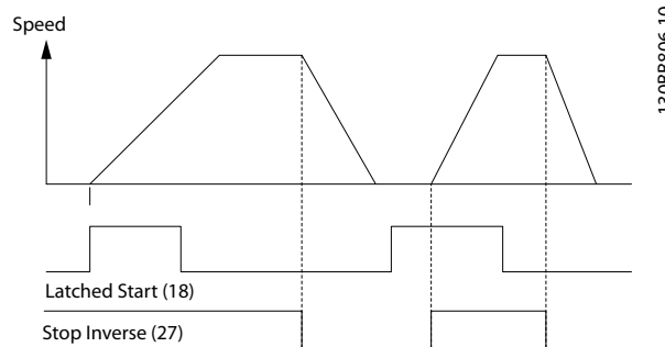
Afbeelding 6.3 Pulsstart/Stop geïnverteerd
