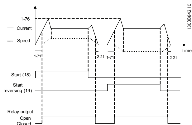
Afbeelding 6.4 Mechanische rembesturing
