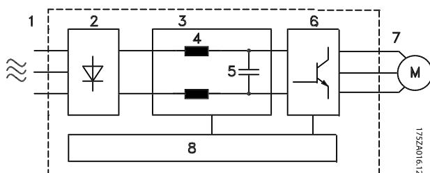
Afbeelding 1.1 Blokschema frequentieomvormer
