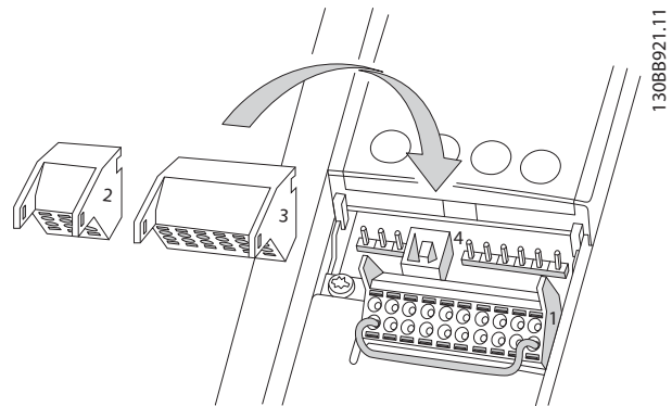
Afbeelding 4.10 Stuurklemposities
