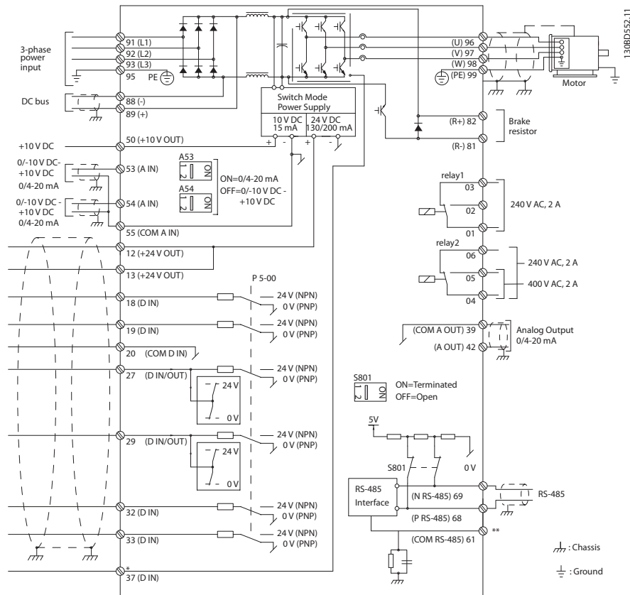
Afbeelding 4.1 Eenvoudig bedradingsschema
