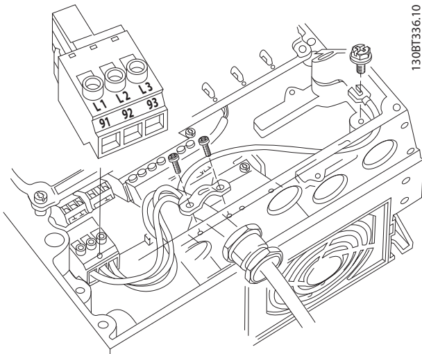
Afbeelding 4.9 Netvoeding aansluiten
