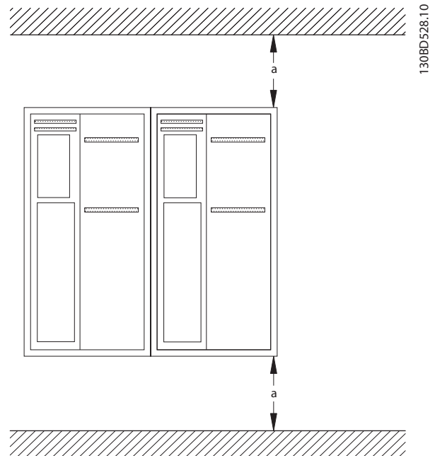
Afbeelding 3.4 Vrije ruimte boven en onder voor luchtkoeling
