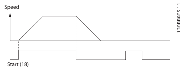
Afbeelding 6.2 Start/stopcommando met Veilige Stop
